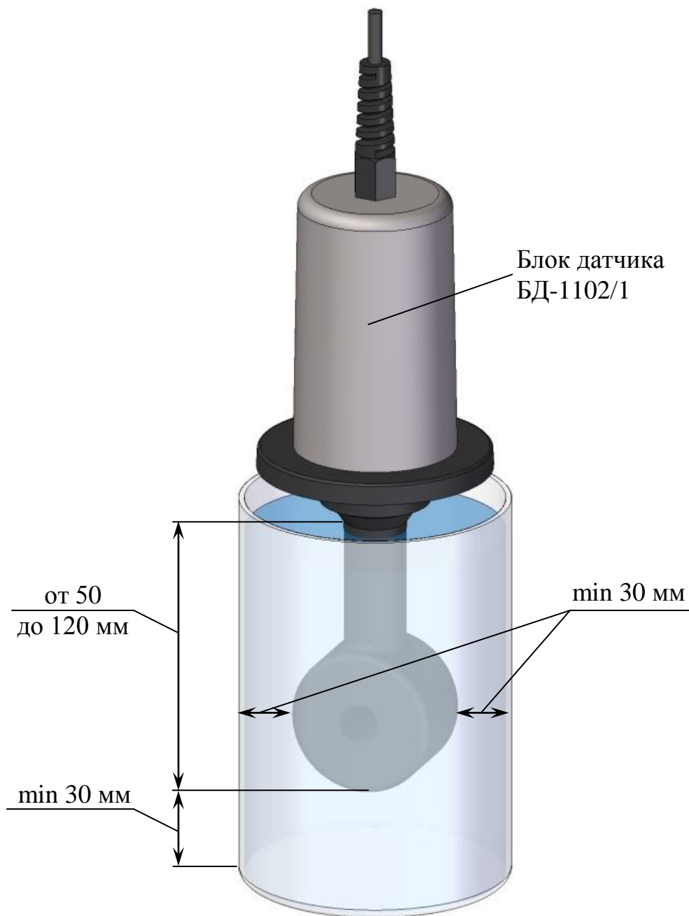
Рисунок 2.15 – Расположение блока датчика БД-1102/1 при проведении измерений погружным способом
