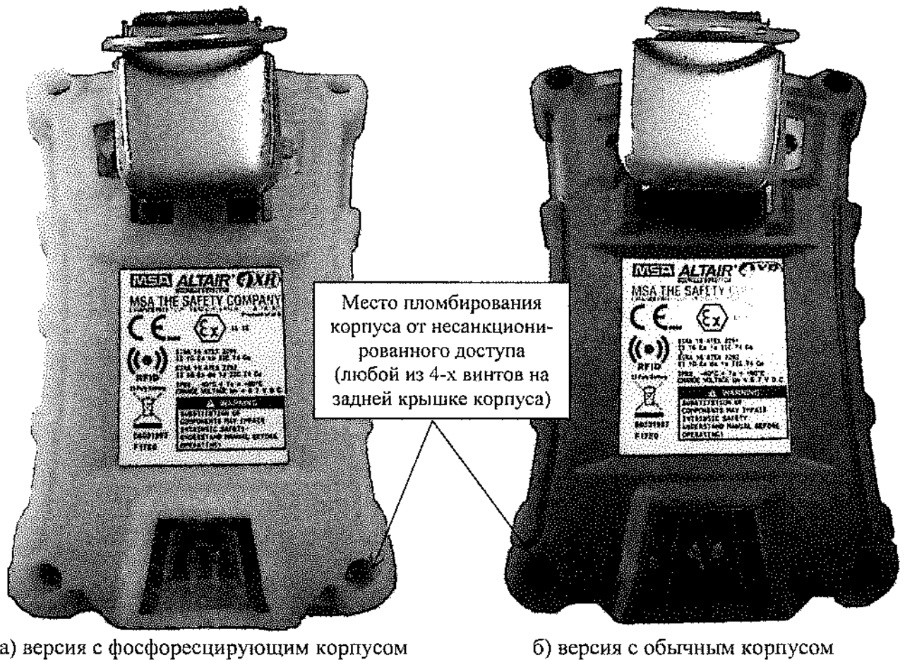
Рисунок 2 - Схема пломбировки корпуса газоанализаторов от несанкционированного доступа
